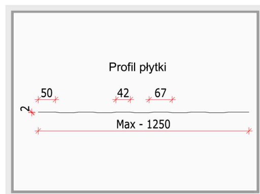
profil płytki
