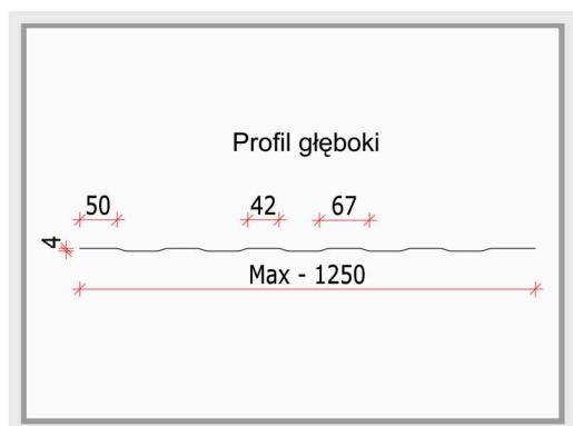
profil głęboki
