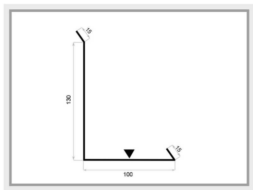
OBD-8 obróbka kominowa
