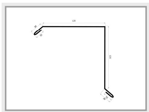
OBD-3 obróbka boczna
