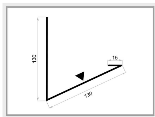
OBD-4 obróbka kominowa 2
