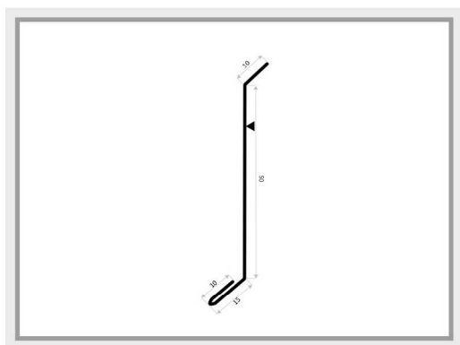
OBD-5 listwa kominowa
