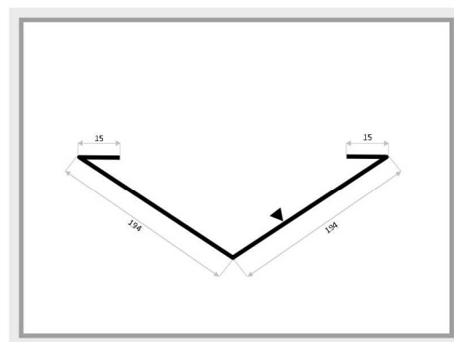
boczna OBD-7 obróbka koszowa
