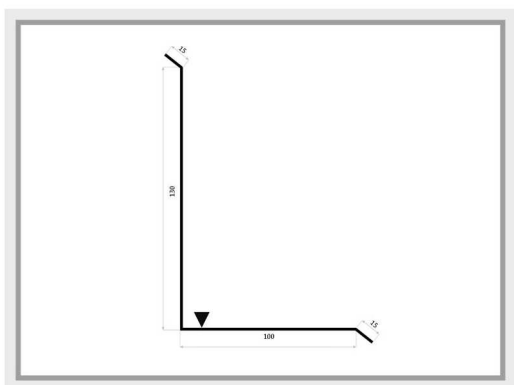
OBD-6 obróbka kominowa
