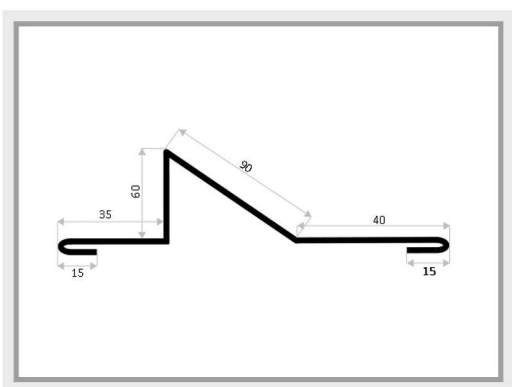
OBP-11 listwa śniegowa
