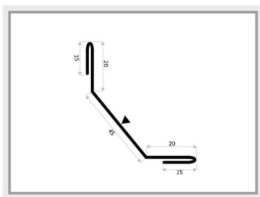
OBP-4 obróbka kątowa skośna
