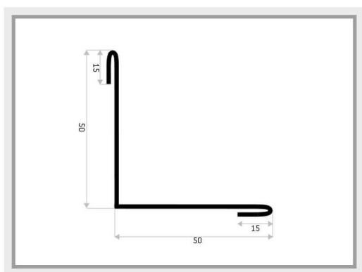
OBP-3 obróbka kątowa wewnętrzna
