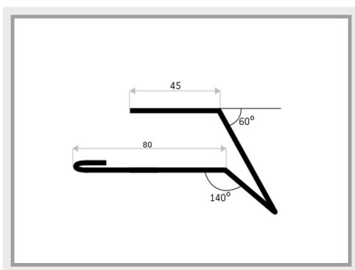
OBP-12 okapnik zam.
