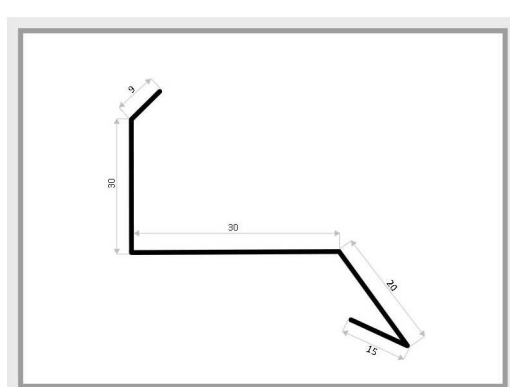
OBP-8 okapnik nad okno
