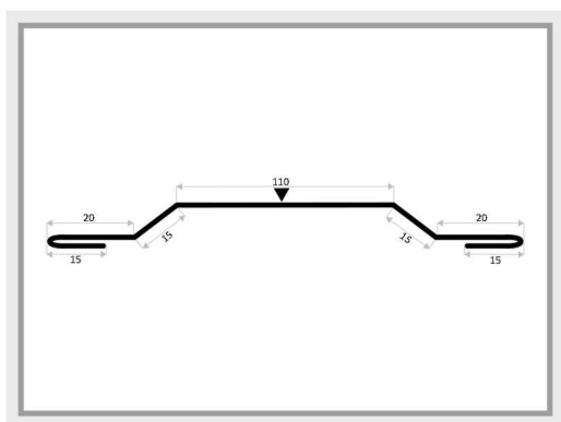
OBP-5 listwa maskująca
