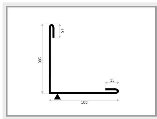
OBP-2 obróbka kątowa zewnętrzna
