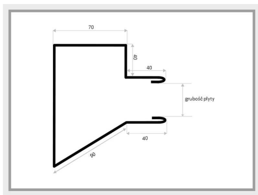
OBP-9 Obróbka boczna zamykająca
