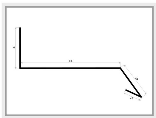
OBP-7 obróbka startowa
