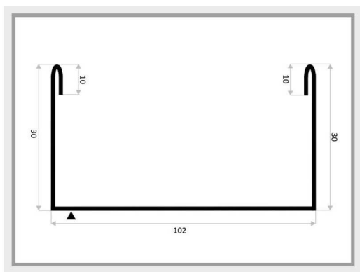
OBP-1 ceownik zakający płytę
